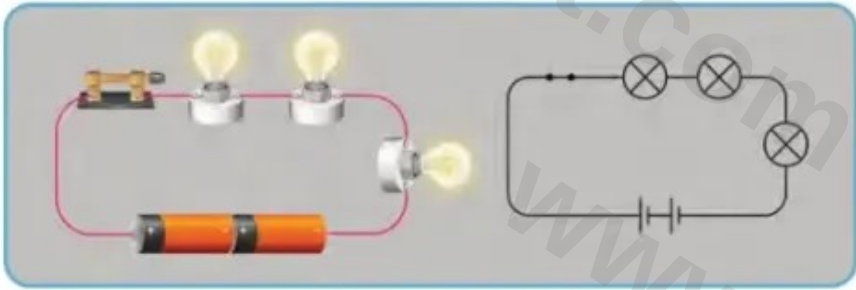
Görsel 6.1.8: Elektrik devre ve şeması
